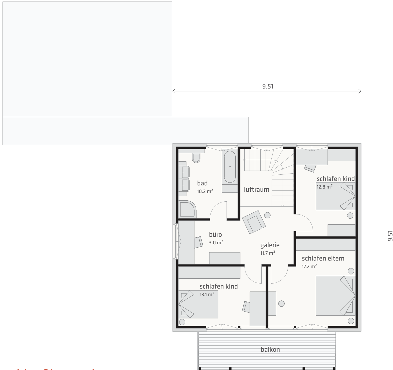
Standardgrundriss Obergeschoss
